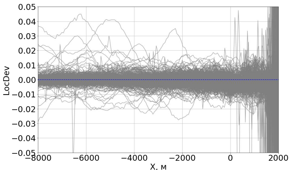
Рисунок 3 – Кривые отклонений самолета от равносигнальной зоны курсового радиомаяка
