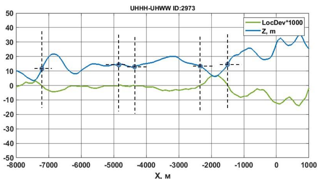
Рисунок 4 – Сопоставление восстановленной траектории и величины отклонения самолета от равносигнальной зоны курсового радиомаяка.
