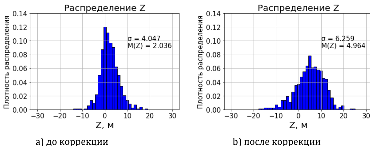
Рисунок 6 – Распределение по Z над торцом ВПП до и после коррекции траекторий (606 траекторий).
