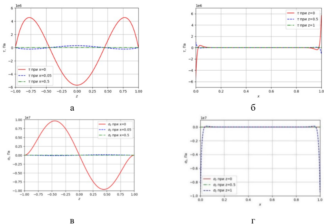
Рис. 2. Компоненты напряжений, вычисленные во втором приближении: а – касательные напряжения \tau_{(2)} в поперечных сечениях; б – касательные напряжения \tau_{(2)} в продольных сечениях; в – поперечные нормальные напряжения \sigma_{z(2)} в поперечных сечениях; г – поперечные нормальные напряжения \sigma_{z(2)} в продольных сечениях
