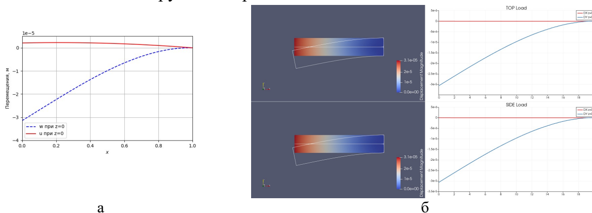
Рис. 13. Перемещения точек полосы в среднем продольном сечении: а – аналитическое решение; б – численное решение, полученное для моделей МКЭ1(вверху) и МКЭ2(внизу) с разными условиями закрепления
