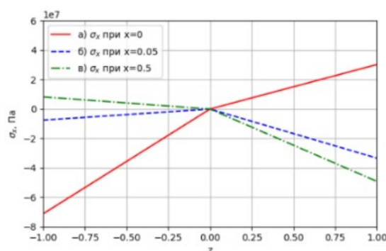
Рис. 7. Распределение напряжений: а – нормальные продольные напряжения [Па] в поперечных сечениях; б – нормальные продольные напряжения [Па] в продольных сечениях
