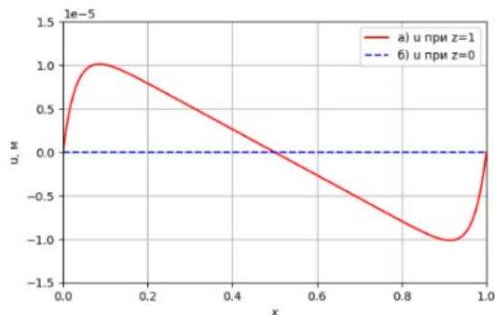
Рис. 5. Продольные перемещения [м] в продольных сечениях
