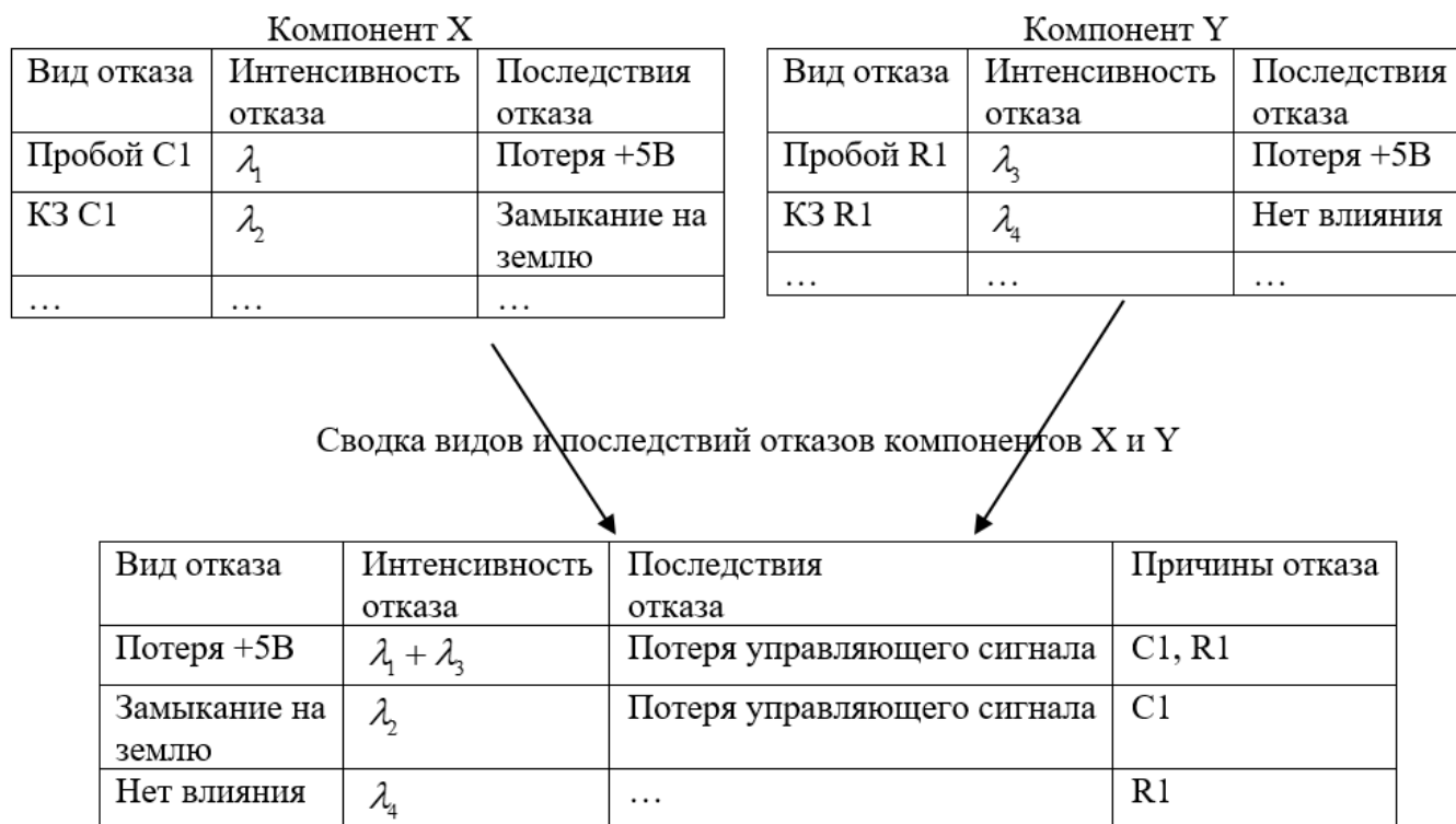
Рисунок 50 Пример перехода от программных и аппаратных АВПО к СВПО
