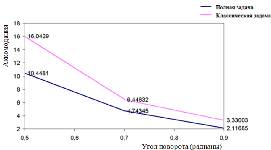
Рисунок 2 - Зависимость коэффициента аккомодации \eta от угла поворота включений относительно оси OX
